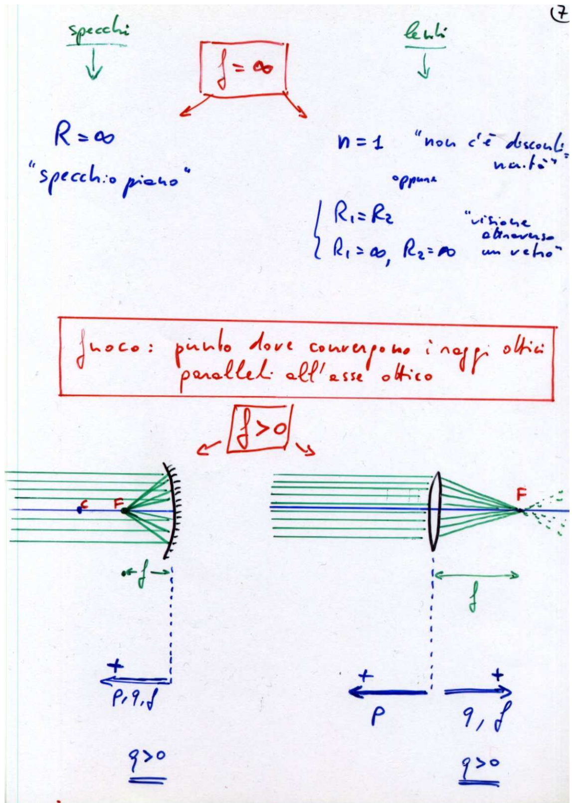
Figura 4.20: Fuochi di specchi e lenti. Convenzione dei segni.
