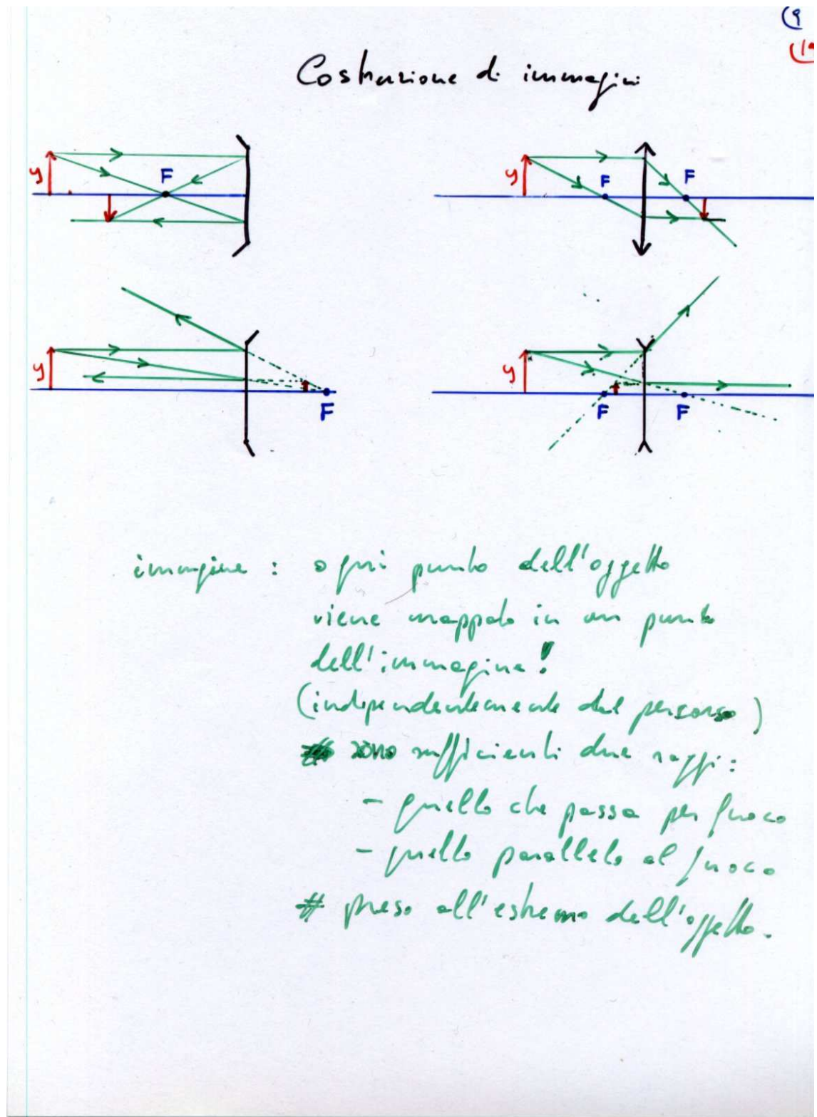
Figura 4.22: Costruzione grafica di immagini.
