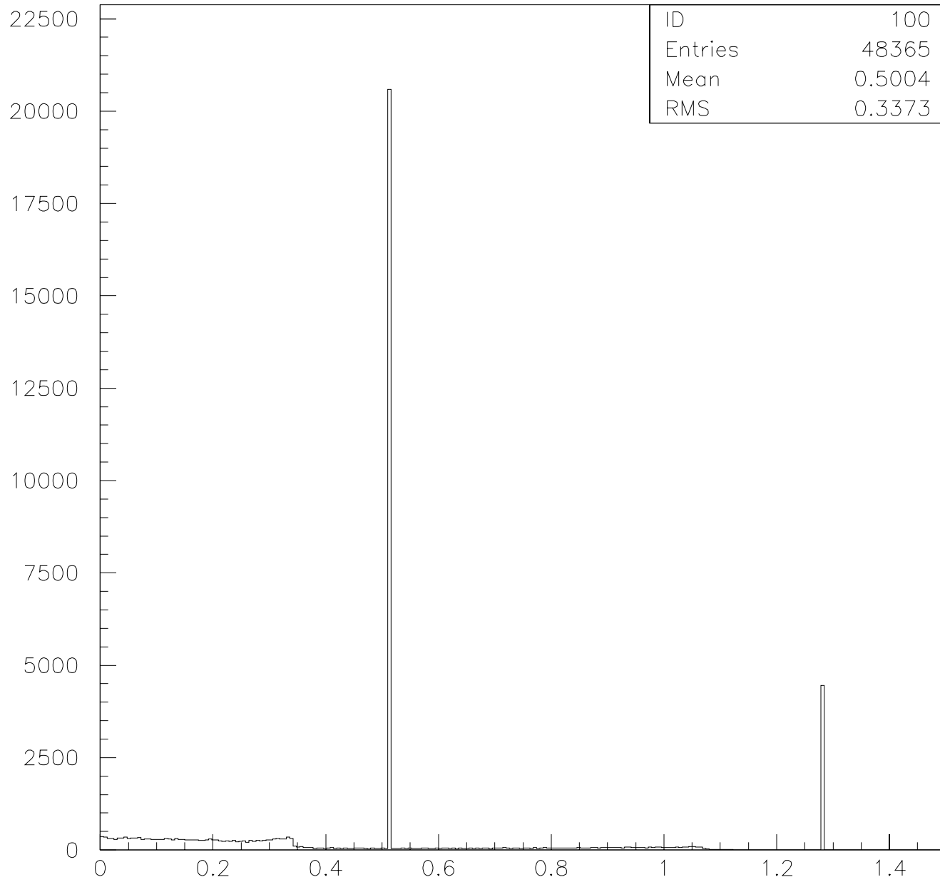
SPETTRO IN ENERGIA SENZA RISOL
