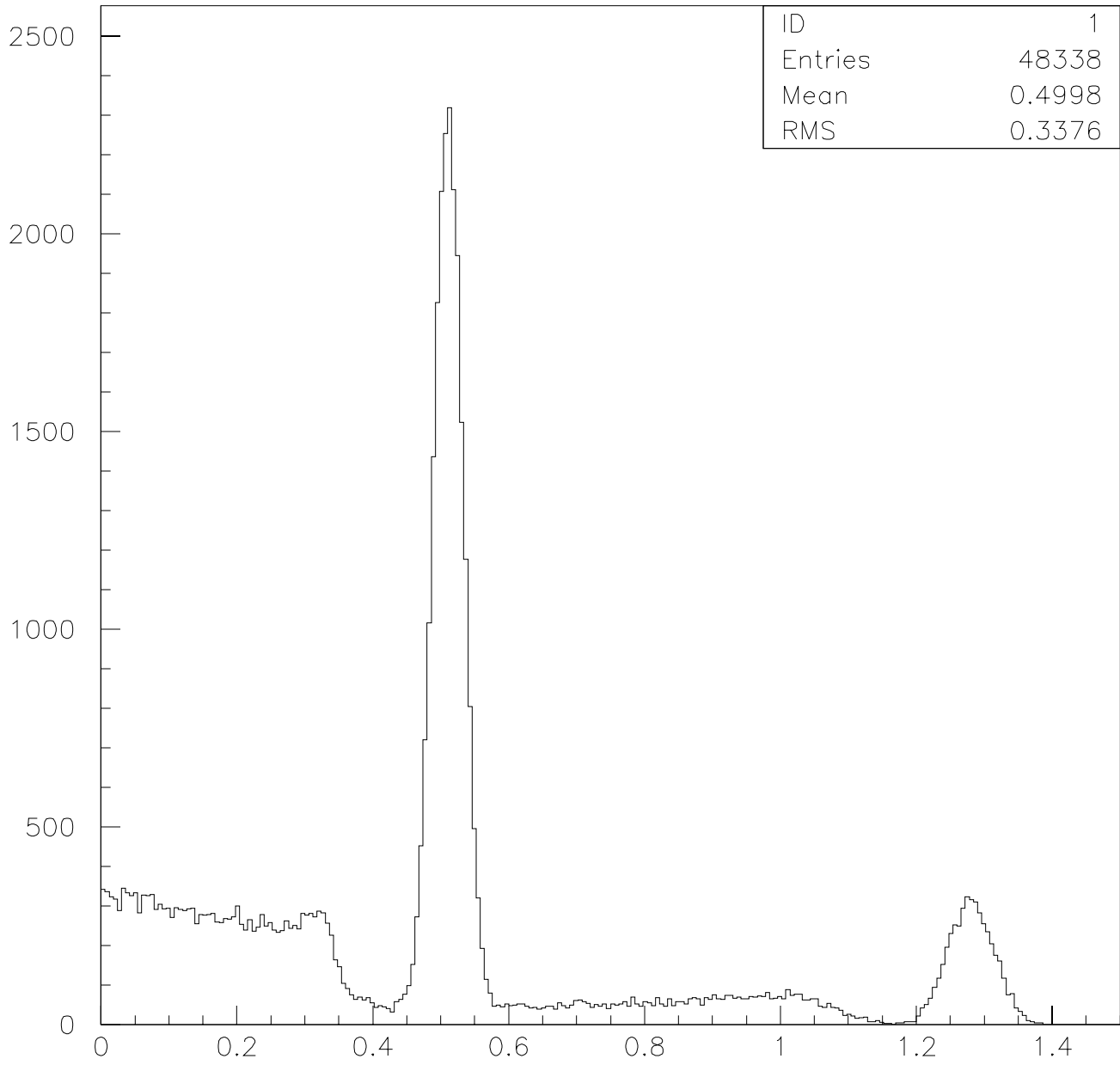
SPETTRO IN ENERGIA
