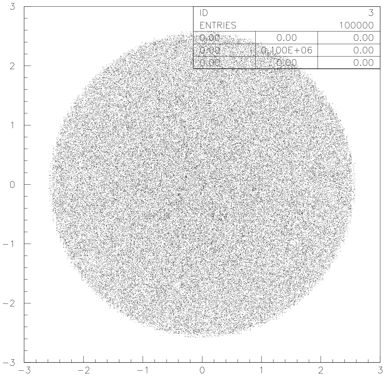
DISTR. PUNTI IMPATTO
