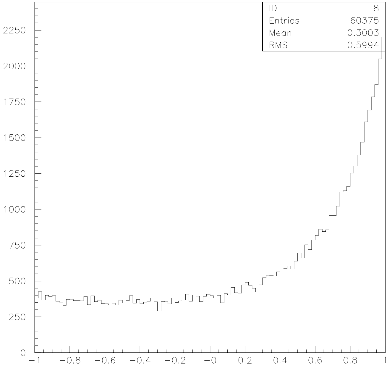
DISTR. COS(TETA) COMPTON
