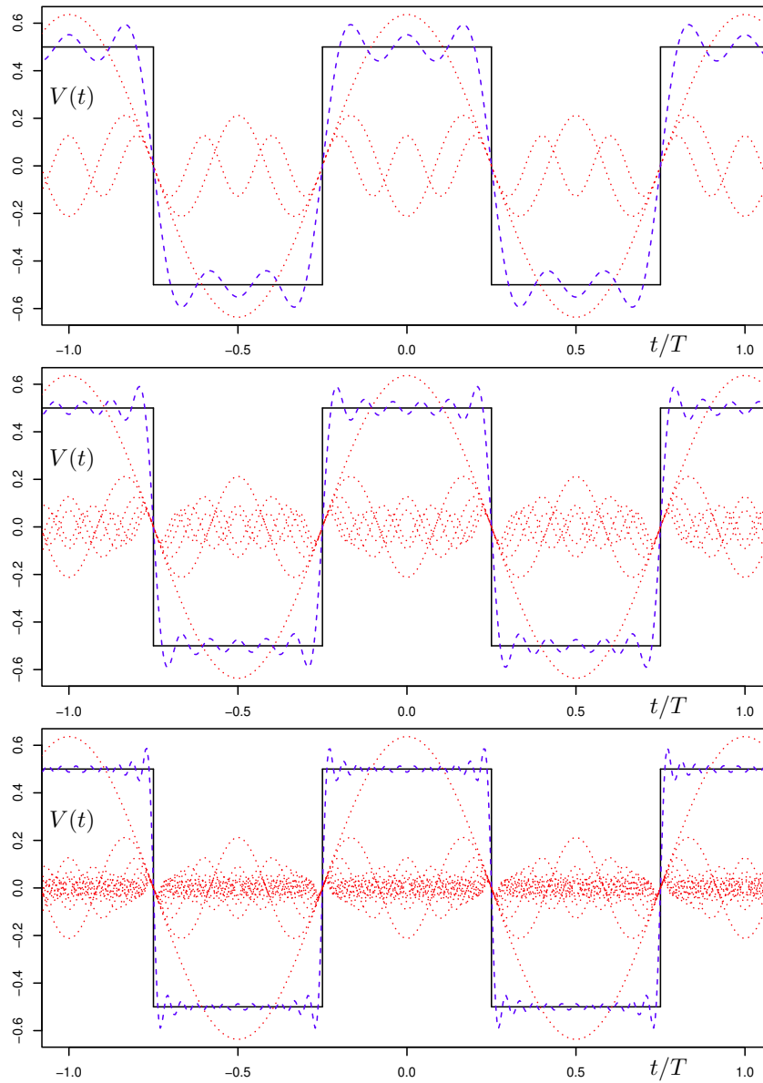
Figura 7.20: Scomposizione in serie di Fourier di un'onda quadra bipolare all'aumentare delle componenti prese in considerazione (dall'alto verso il basso): prime 3, prime 6 e prime 12.
