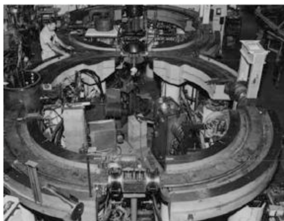
Il collider a doppio anello elettrone-elettrone da 500 MeV costruito a Stanford a partire dal 1959. I risultati sulla verifica dell'elettrodinamica furono pubblicati solo nel 1966.
